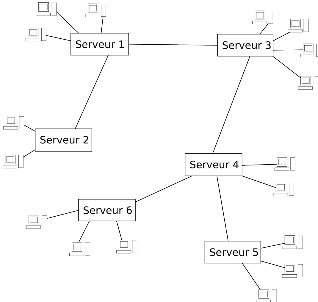
Illustration 14: Internet Relay Chat : Exemple d'un réseau IRC distribué
