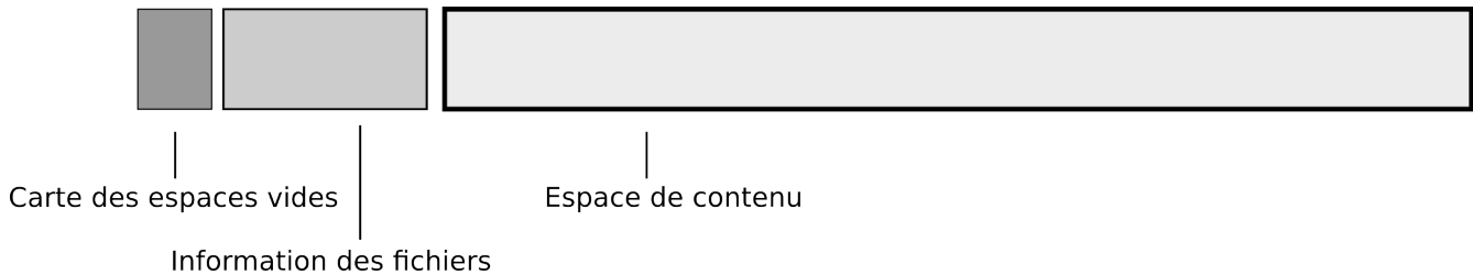
Illustration 10: Système de fichiers : Trois grandes sections d'un disque dur
