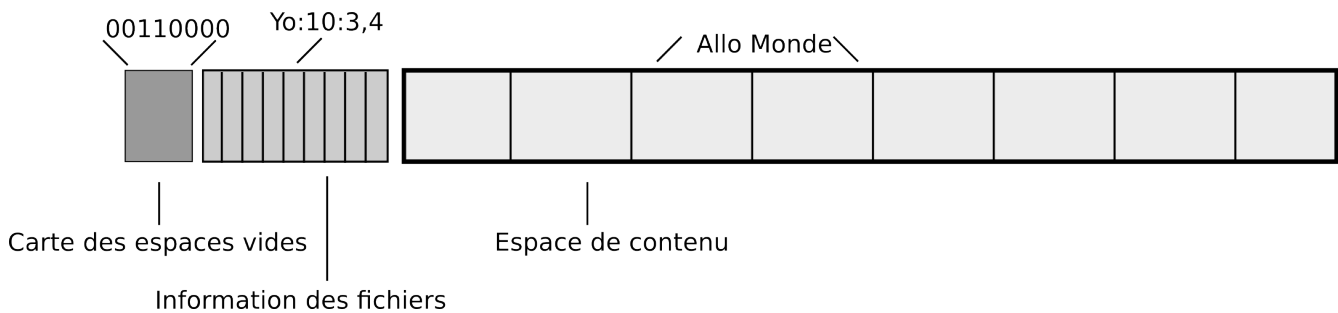
Illustration 11: Système de fichiers : Exemple des trois sections avec un "Allo Monde"
