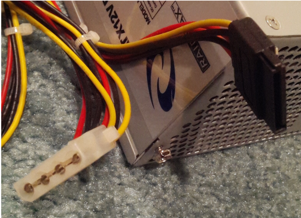
Illustration 7: Les composantes d'un ordinateur : Câble alimentation IDE (blanc) et SATA (noir)
