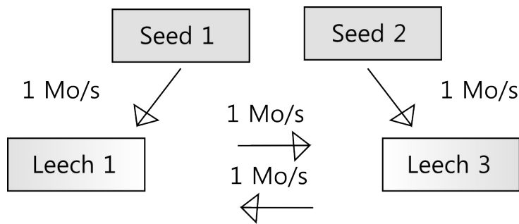
Illustration 20: BitTorrent : Transfert de fichier avec BitTorrent (2 seeder et 2 leechers)
