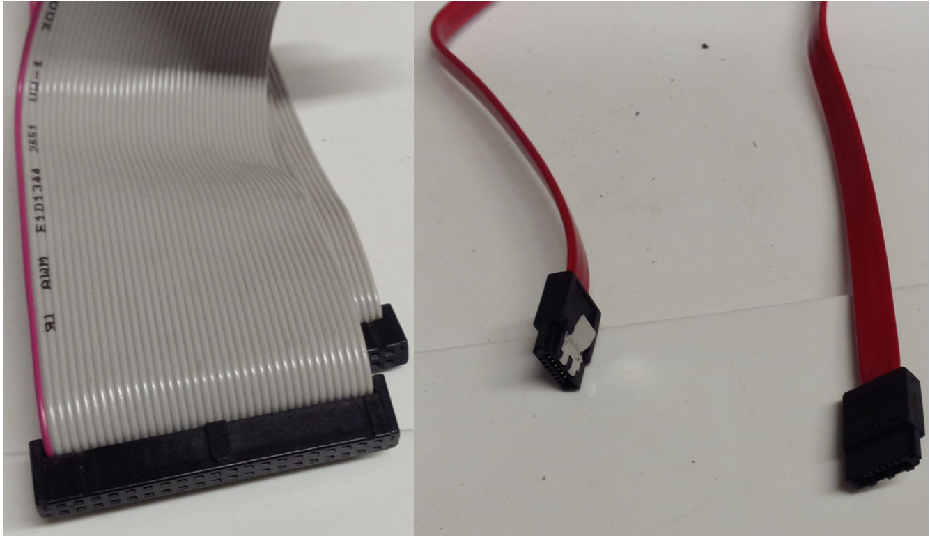
Illustration 6: Les composantes d'un ordinateur : Câble IDE à gauche et câble SATA à droite
