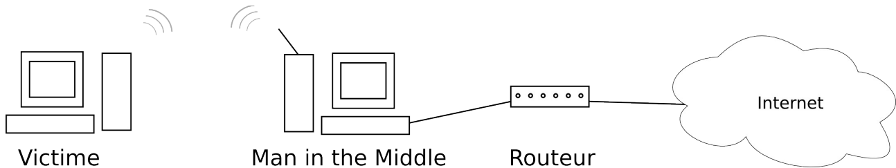
Illustration 22: Insécurité d'Internet : Attaque de l'homme au milieu à l'aide d'une borne WiFi
