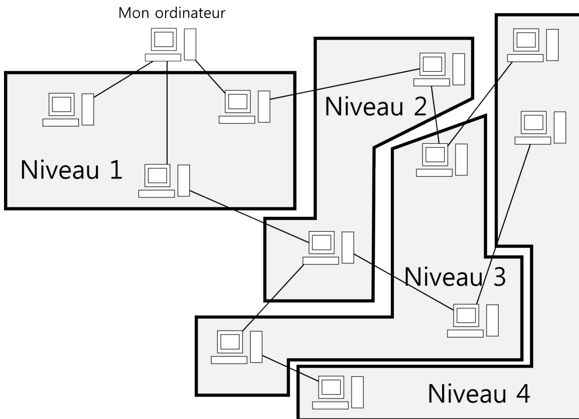
Illustration 16: Gnutella : Propagation des messages sur Gnutella
