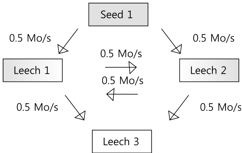
Illustration 19: BitTorrent : Transfert de fichier avec BitTorrent (1 seeder et 3 leechers)
