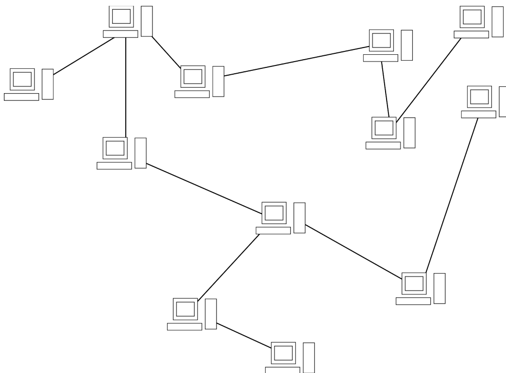
Illustration 15: Gnutella : Exemple de réseau Gnutella décentralisé
