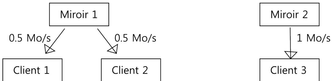
Illustration 17: BitTorrent : Transfert de fichier normal avec l'utilisation de miroirs
