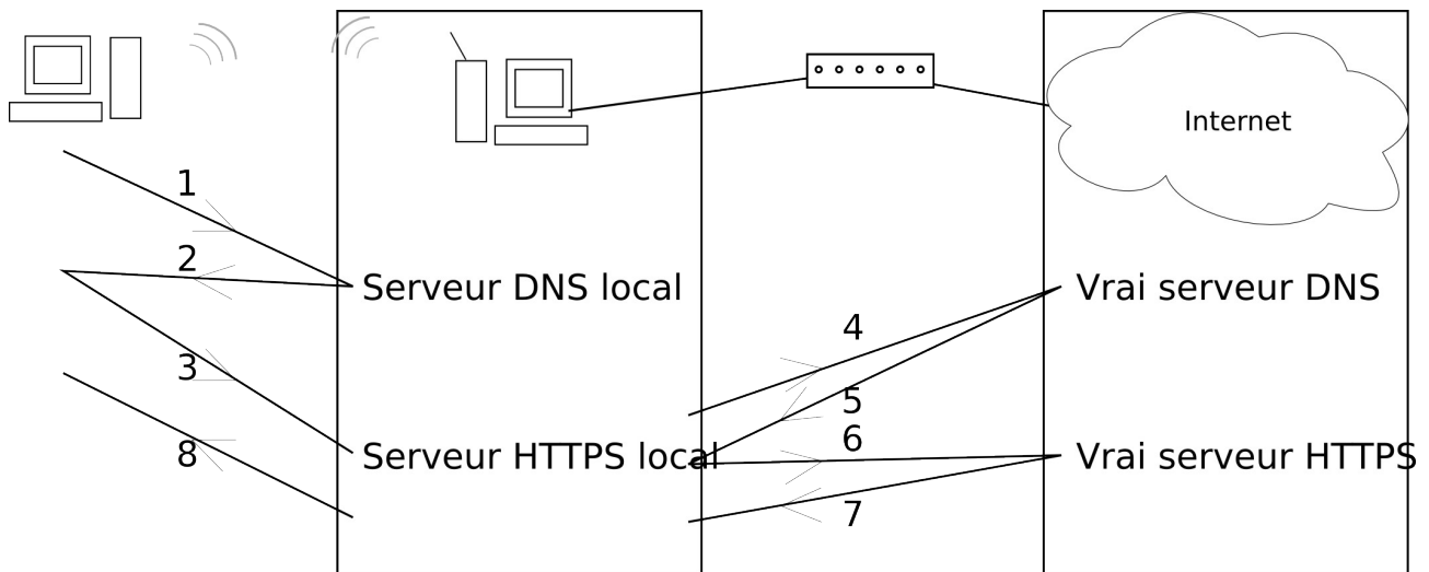
Illustration 24: Insécurité d'Internet : Attaque de l'homme au milieu qui voit le HTTPS
