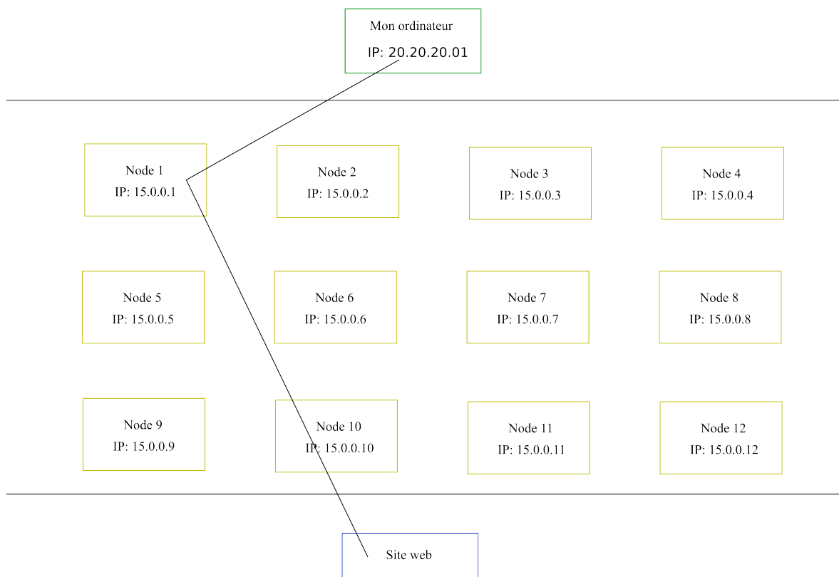
Illustration 25: Tor : Route sur Tor
